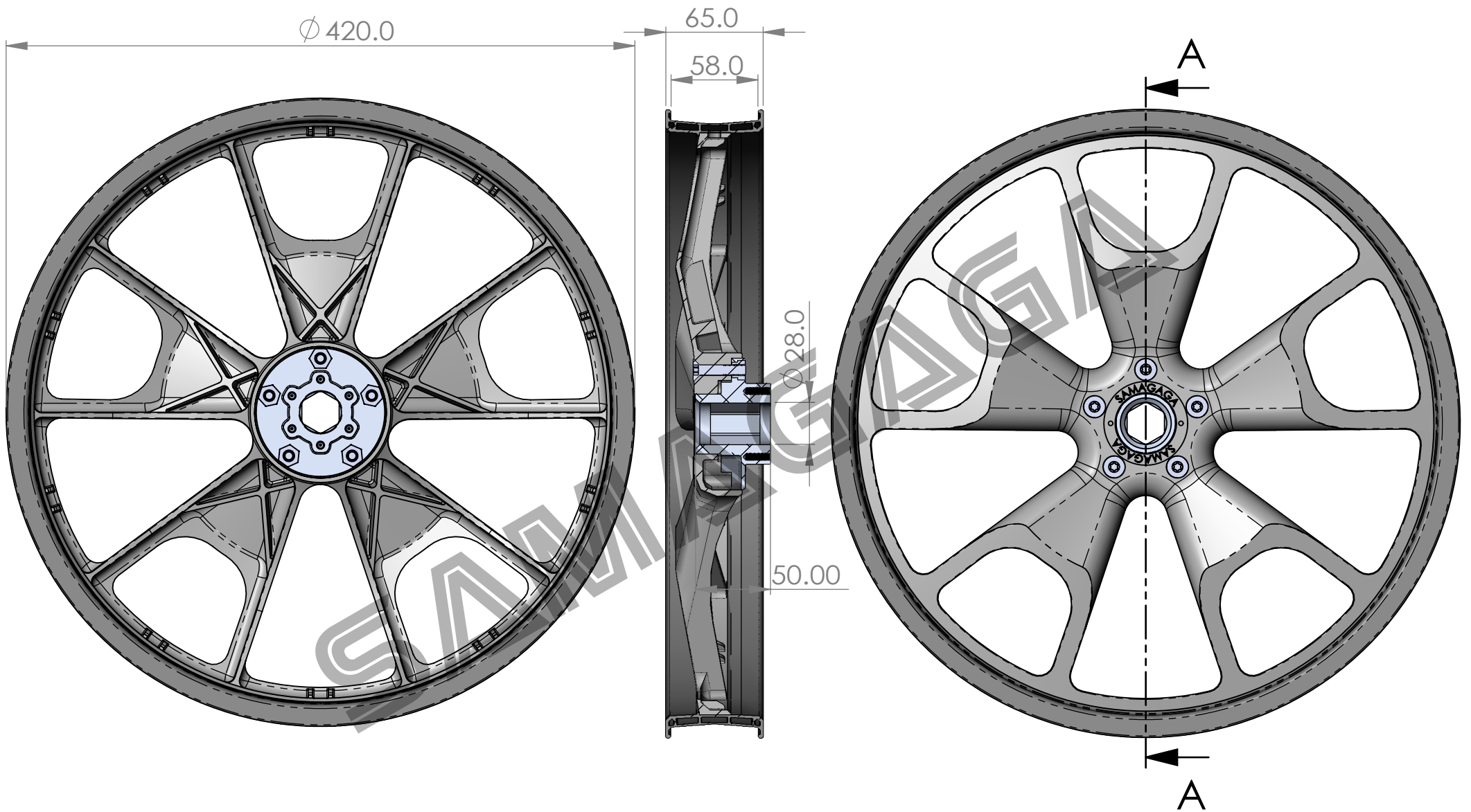
剖面圖 A-A
